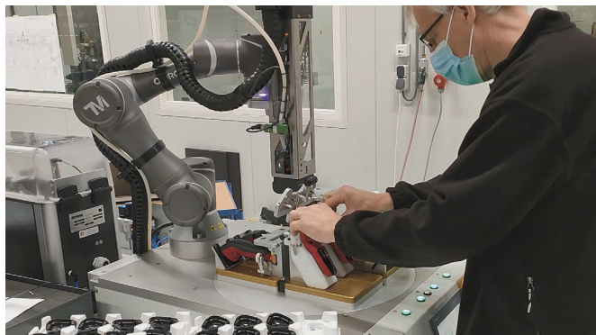
協調ロボットと人が共同で組立作業を行う様子
